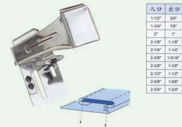
JZ-15536 F201 门襟筒 Top Center Plait Folder
