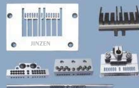
1412P 13N 1/8 13N 3/16 13N 1/4 JZ-12107
