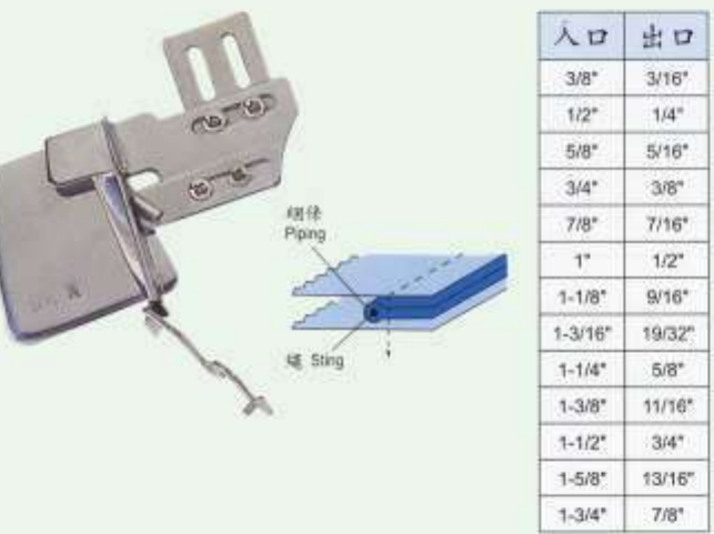
JZ-15535 F521 活动绳子筒 Piping Folder
